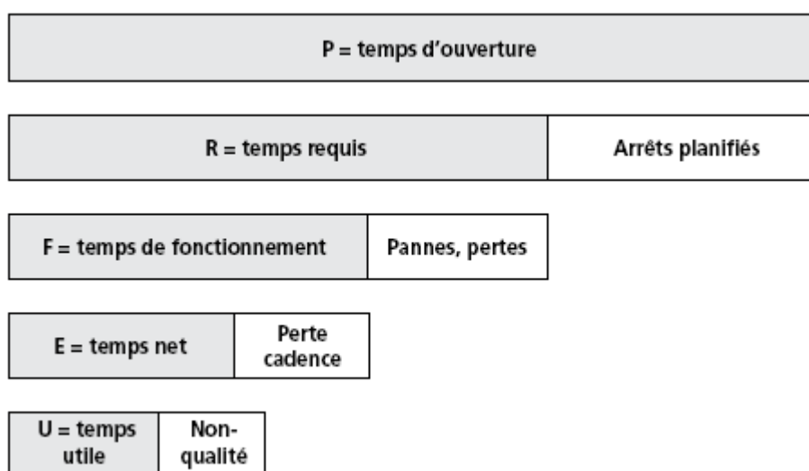
Figure 8 Principe de découpage analyse TPM
