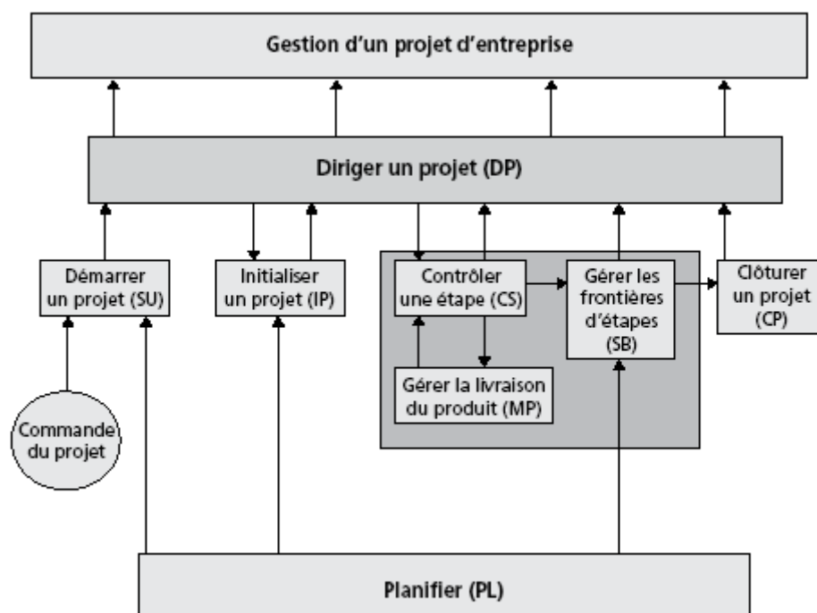
Figure 4 Modèle PRINCE2
