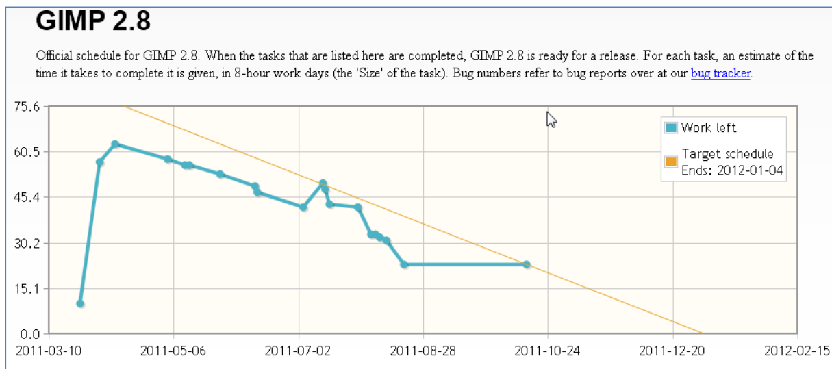
Figure 37 Extrapolation linéaire du groupe de développement du logiciel GIMP
