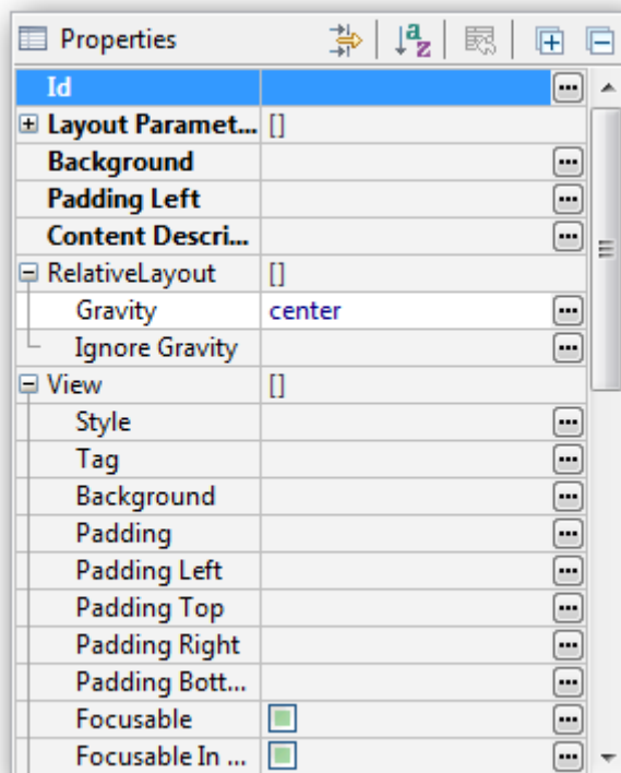
Figure 3.7 – L'encart « Properties »
