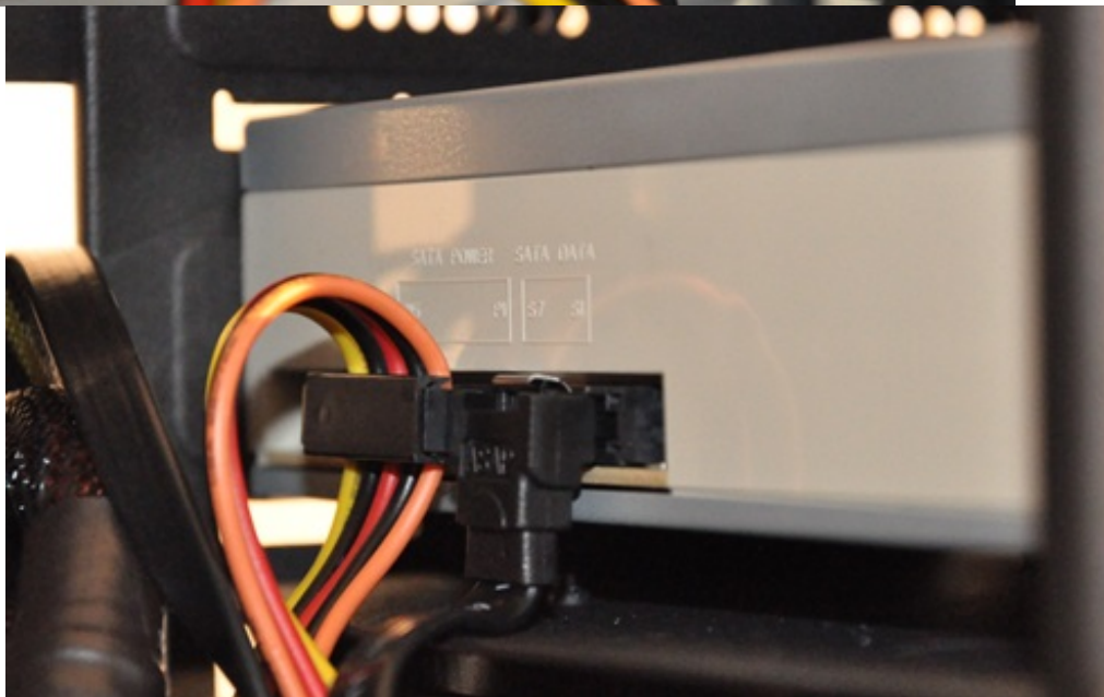
du lecteur-graveur en SATA
