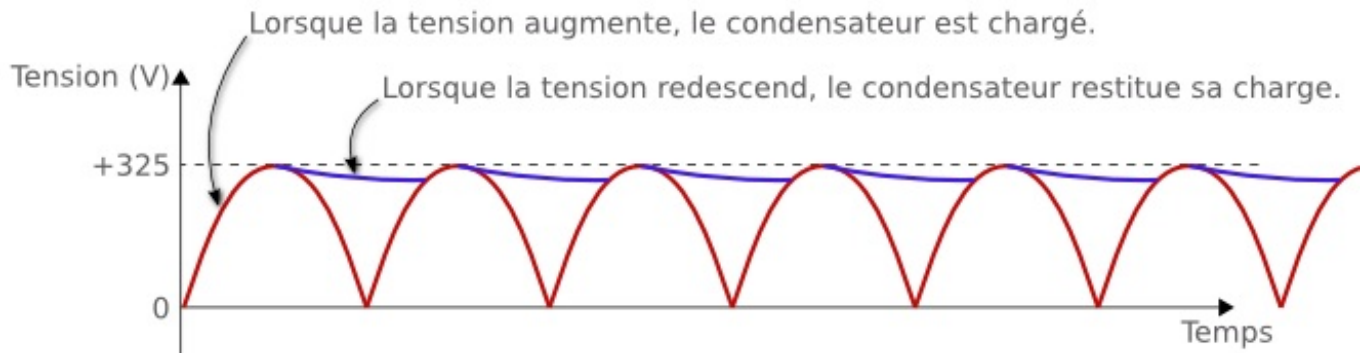
Charge et décharge d'un condensateur pour lisser une tension
