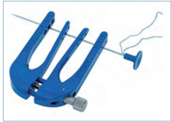
32.11 Appareil Achillon® pour suture mini-invasive.
