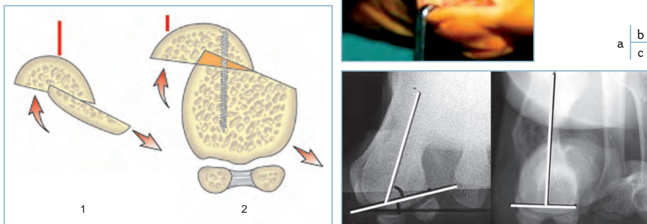
6.52 Rotation axiale : en avant, résection médiale ; en arrière, l'effet de tuile est bénéfique. a. Représentation schématique d'une ostéotomie supinante. Enclavement proximal (I), résection cunéiforme et supination distale de la tête (2). b. Vue peropératoire. c. Réorientation en vue axiale objectivant la supination céphalique à l'appui (troisième dimension de la correction).
