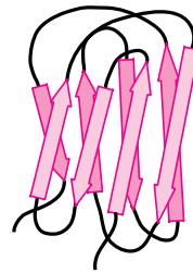
Domaine \beta
