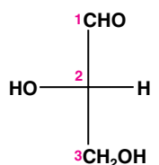
L-Glycéraldéhyde
