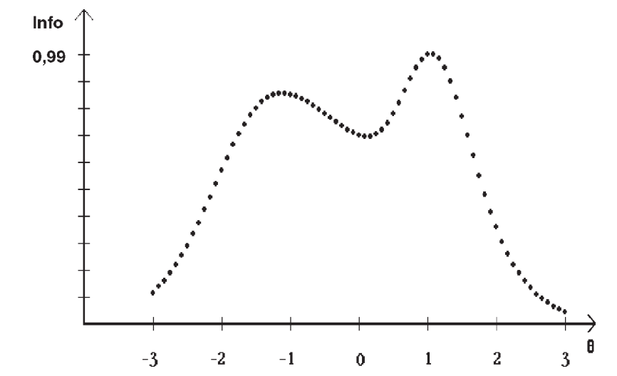
FIGURE 4.31 Courbe d'information d'un test de 4 items
