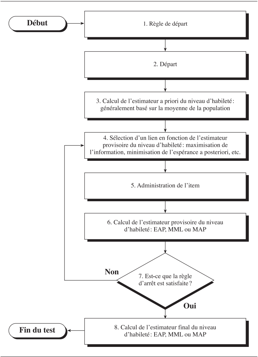
FIGURE 9.2 Structure d'un test adaptatif basé sur la théorie des réponses aux items (d'après Raîche, 2000, p. 71)
