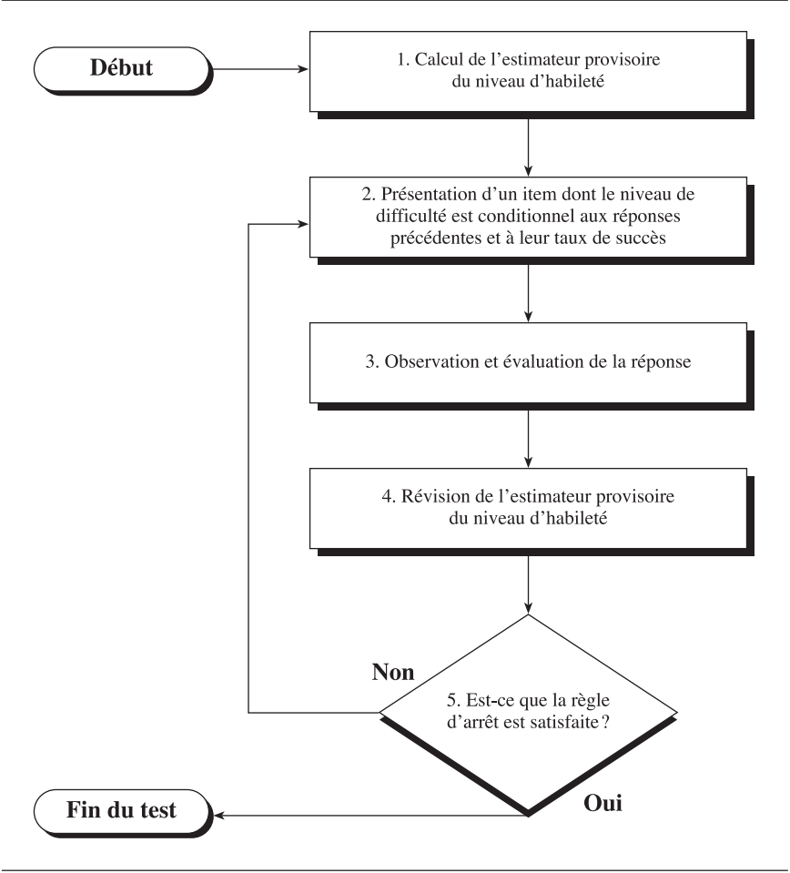
FIGURE 9.1 Déroulement général d'un test adaptatif (d'après Raïche, 2000, p. 22)
