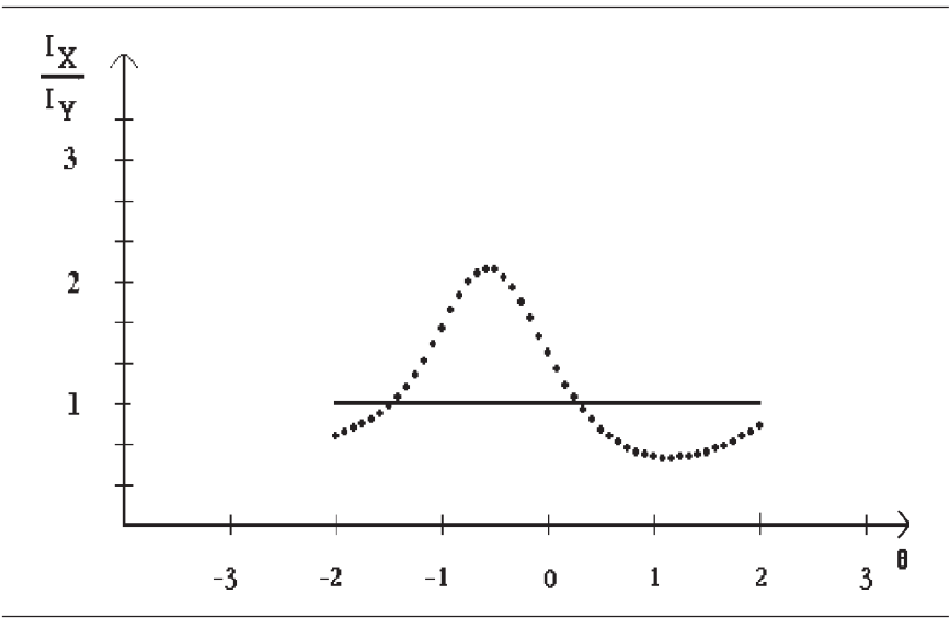
FIGURE 4.34 Efficacité relative de deux tests de 19 items chacun : le test X informe surtout autour de \theta = 0 alors que le test Y informe dans le voisinage de \theta = 1 .
