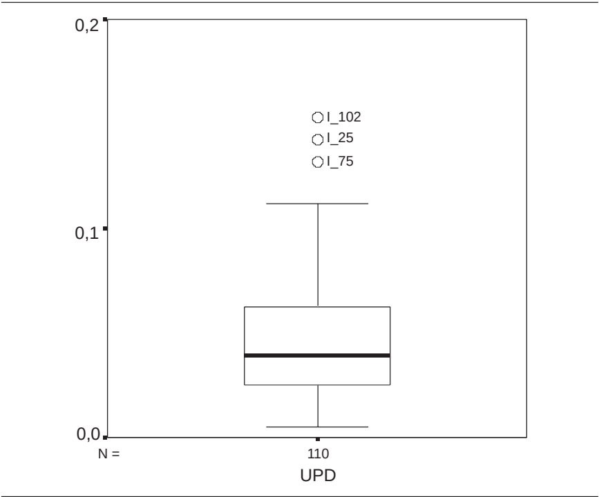
FIGURE 8.8 Diagramme en boîte et moustaches indiquant les valeurs aberrantes (O) de l'indice UPD de Shepard, Camilli et Williams (1984) pour les 110 items de l'enquête du PIRS en 1997.
