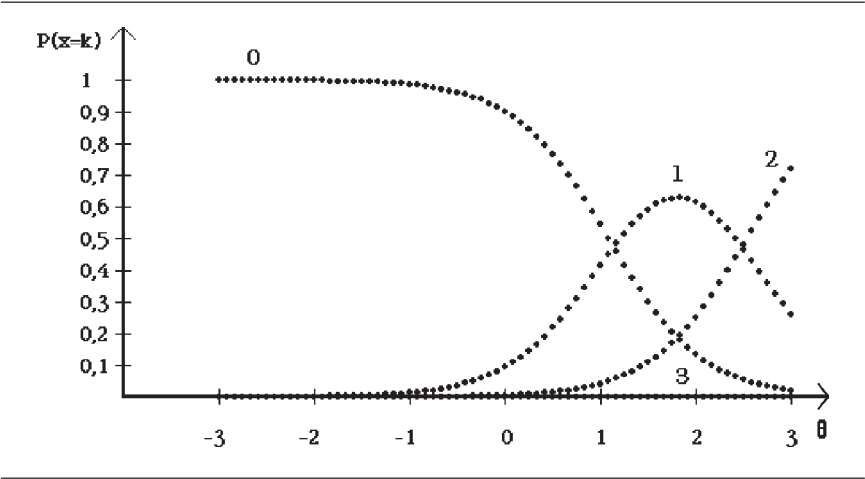
FIGURE 4.37 Courbes caractéristiques de chacune des 4 catégories de l'item 13 de l'échelle de dépression de Beck
