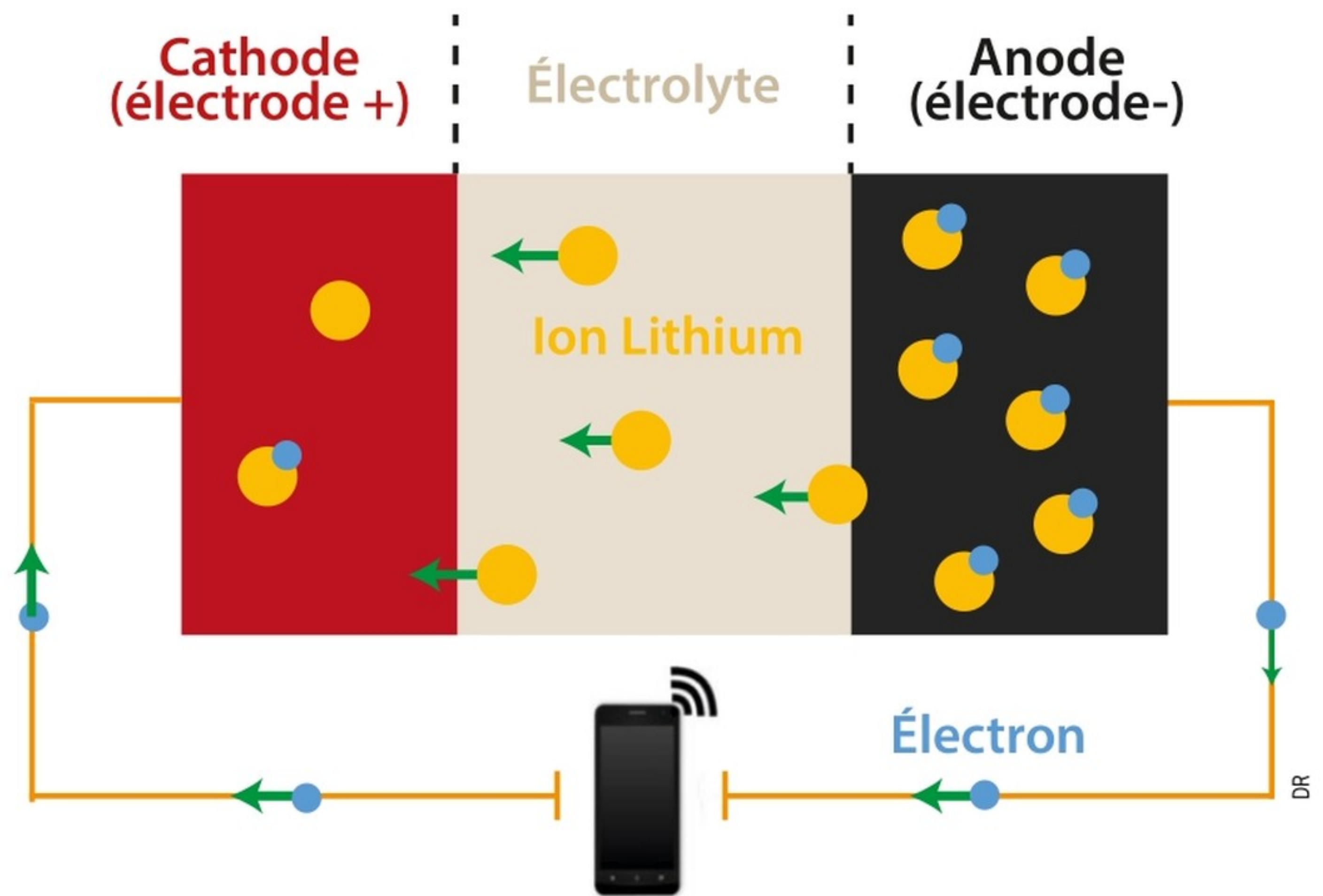
▲ Pour produire l'électricité nécessaire, les électrons passent de l'anode à la cathode par le circuit, et dans le même temps les ions de lithium se déplacent à travers l'électrolyte vers la cathode.
