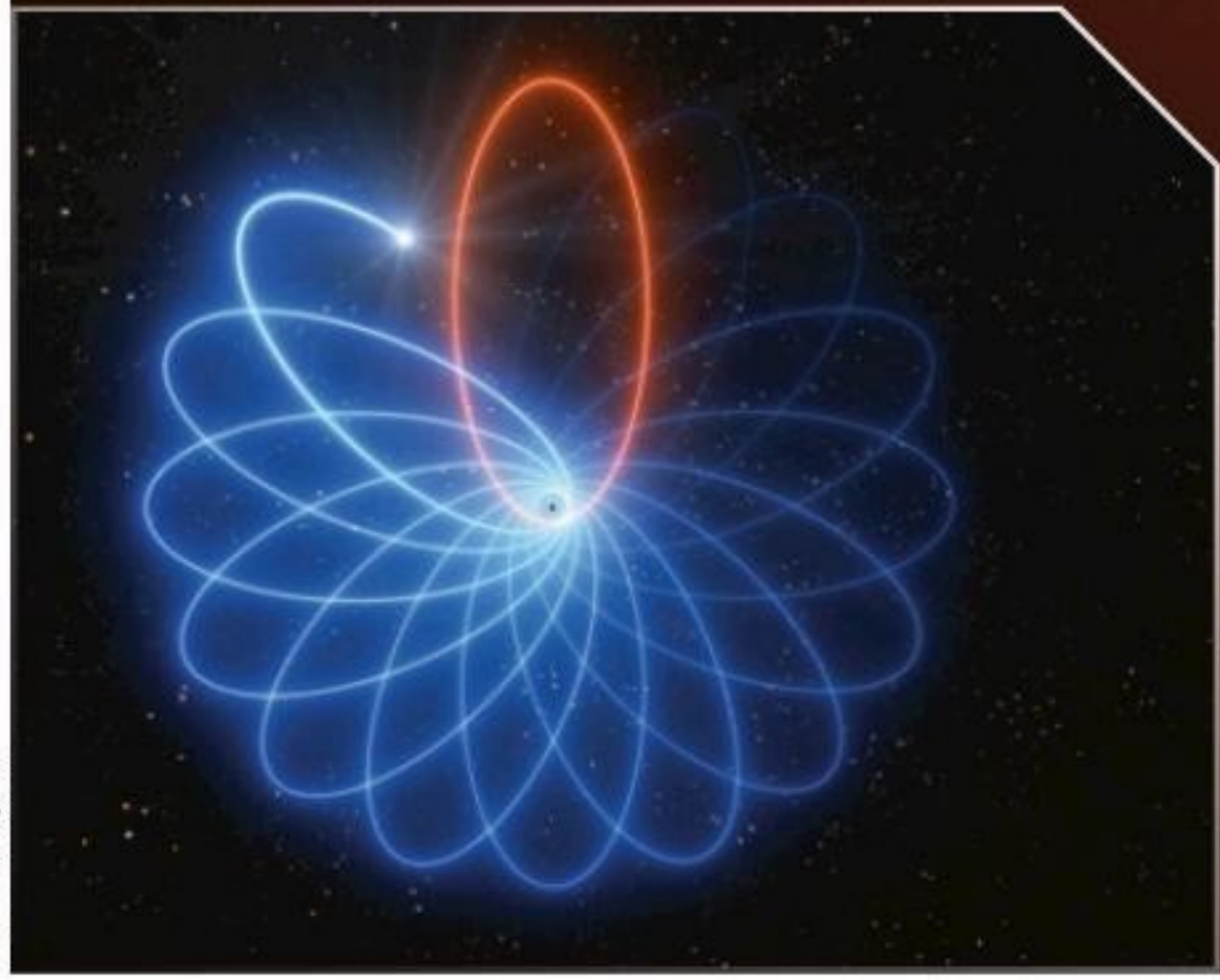
Vue d'artiste (exagérée) de l'orbite d'une étoile autour du trou noir Sagittarius A* (en bleu). Cette trajectoire en rosette valide la relativité générale d'Einstein et non la gravité de Newton, qui prédisait une simple ellipse.
