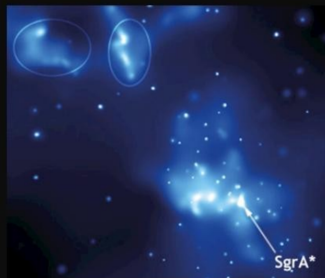
Image aux rayons X de la région autour de Sagittarius A* (Sgr A*), le trou noir trônant au centre de notre Voie lactée.
