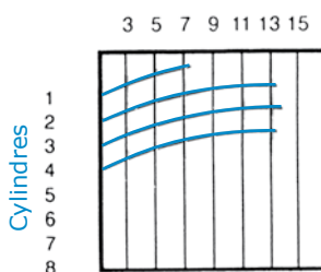
Manque de compression sur cylindre n° 1
