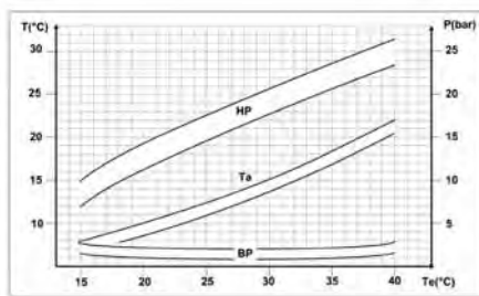
Courbe d'efficacité du système
