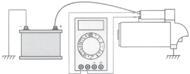
Contrôle du relais de commande
