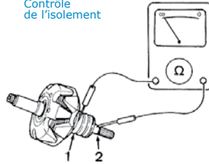
Contrôle du rotor
