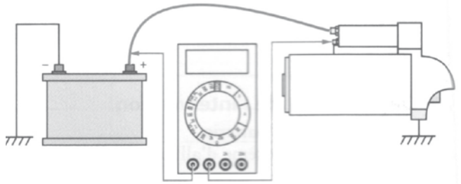
Contrôle du fil d'alimentation
