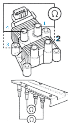
Résistance secondaire sur bobine jumostatique (exemple)
