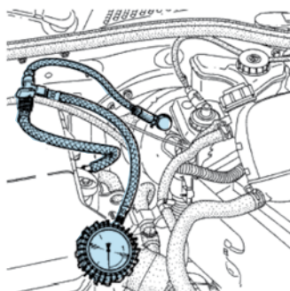
Branchement du manomètre
