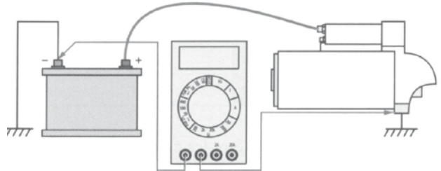
Contrôle de la liaison avec la masse
