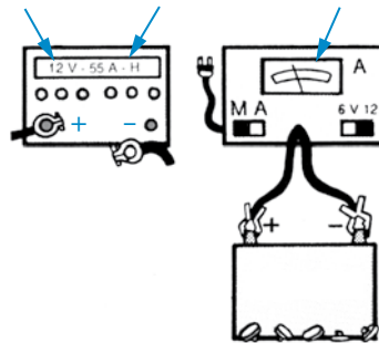
Brancher le chargeur.
