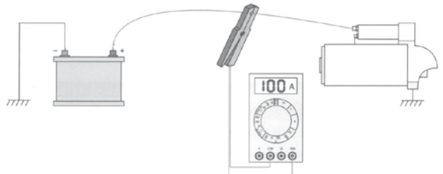
Contrôle de la consommation
