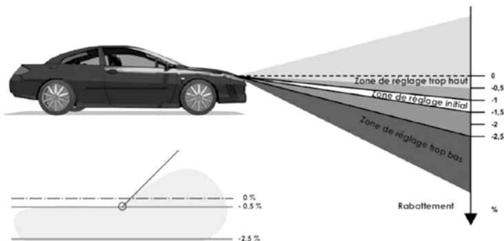
Zone de rabatement de faisceau
