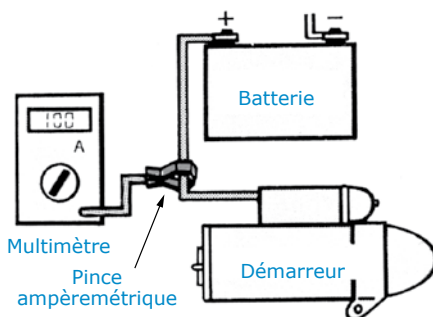
Contrôle de l'intensité de démarrage.
