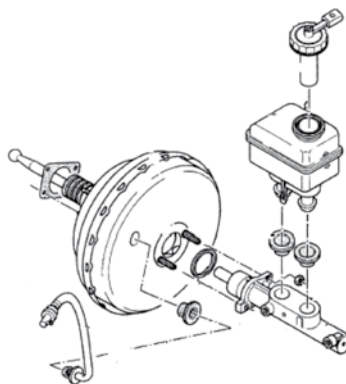
Ampli.cateur de freinage (servo-frein) + maître cylindre
