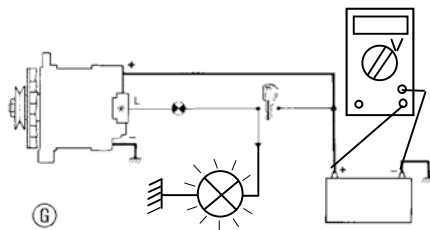
Contrôle de la tension régulée
