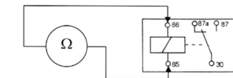
Contrôle circuit de commande
