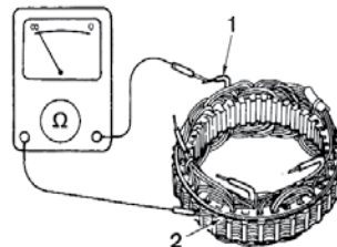
Contrôle du stator
