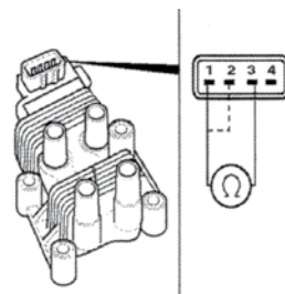
Résistance primaire sur bobine jumostatique (exemple)
