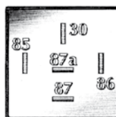
Brochage DIN
