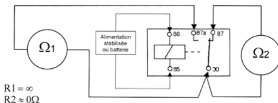
Circuit de puissance contact au travail
