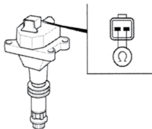
Résistance primaire sur bobine statique (exemple)
