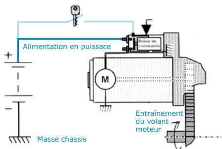
Branchement du démarreur
