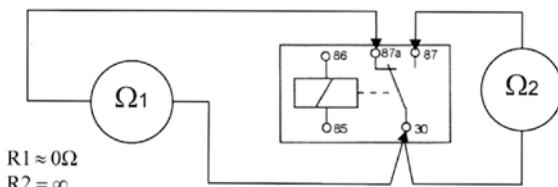
Circuit de puissance contact au repos
