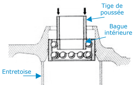
Extraction du roulement de roue
