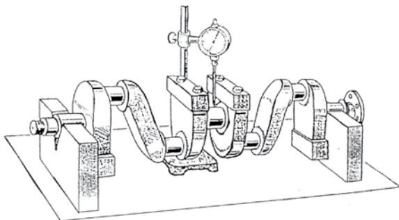
Exemple de réglage de jeu latéral
