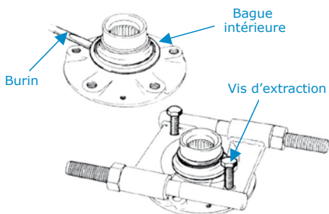
Extraction de la bague intérieure
