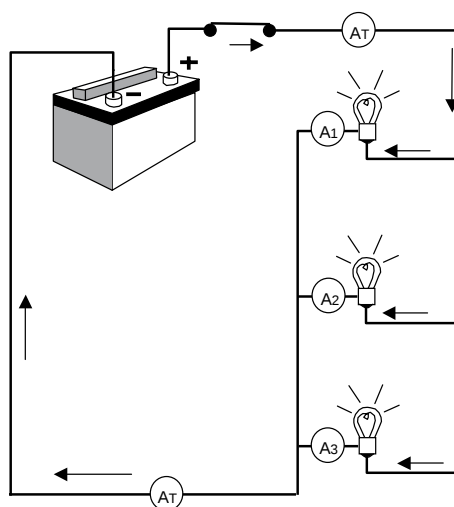
Montage parallèle (dérivation)
