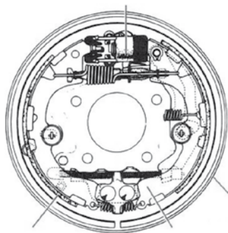
Déposer le tambour
